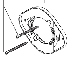
RP100725▲ Escutcheon & Gasket Roseta y Empaque Rosace avec Orifice et Joint
